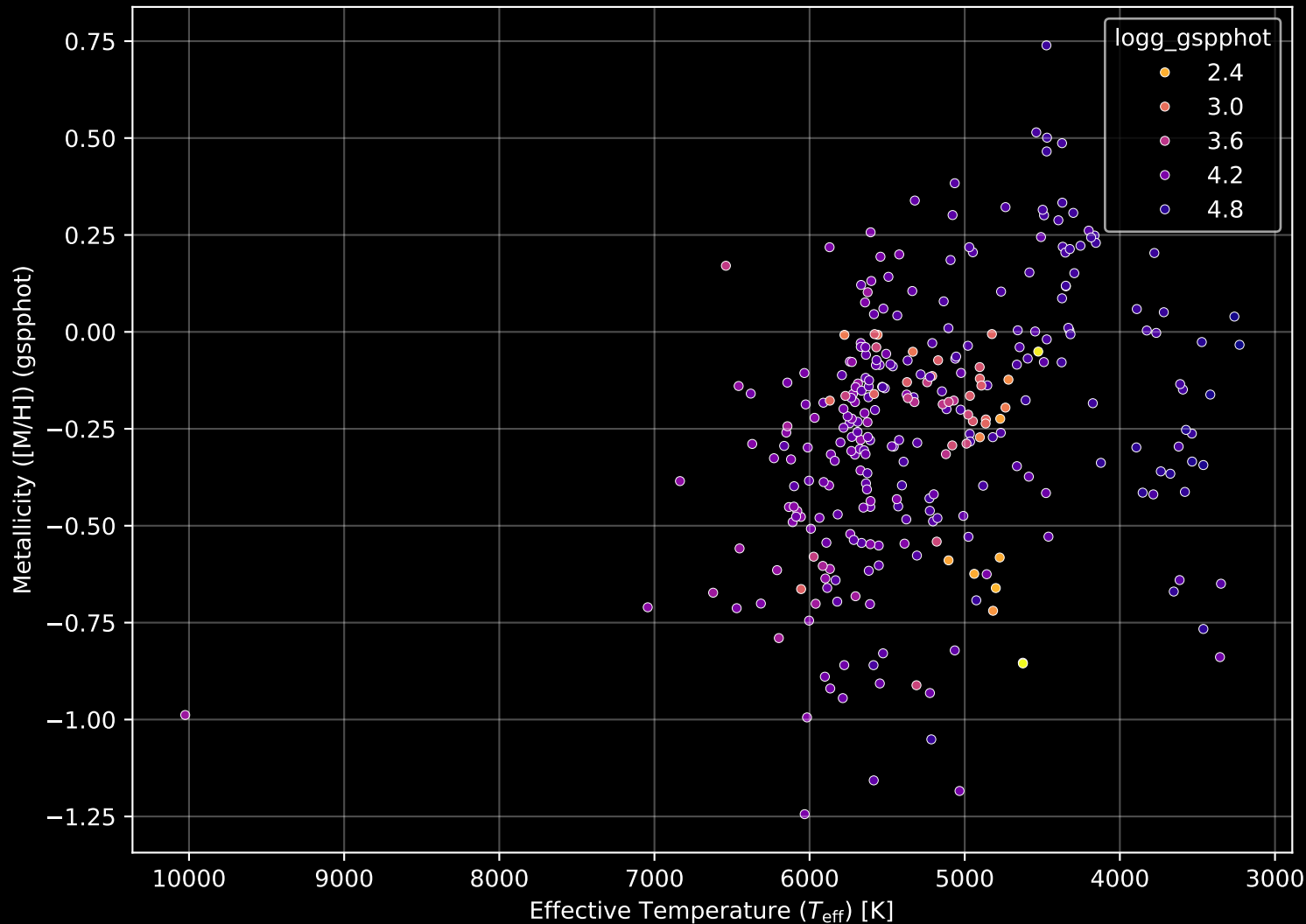
APOGEE DR17 Field: [sgr_tidal8] Stellar Population Parameters (n= 301)
